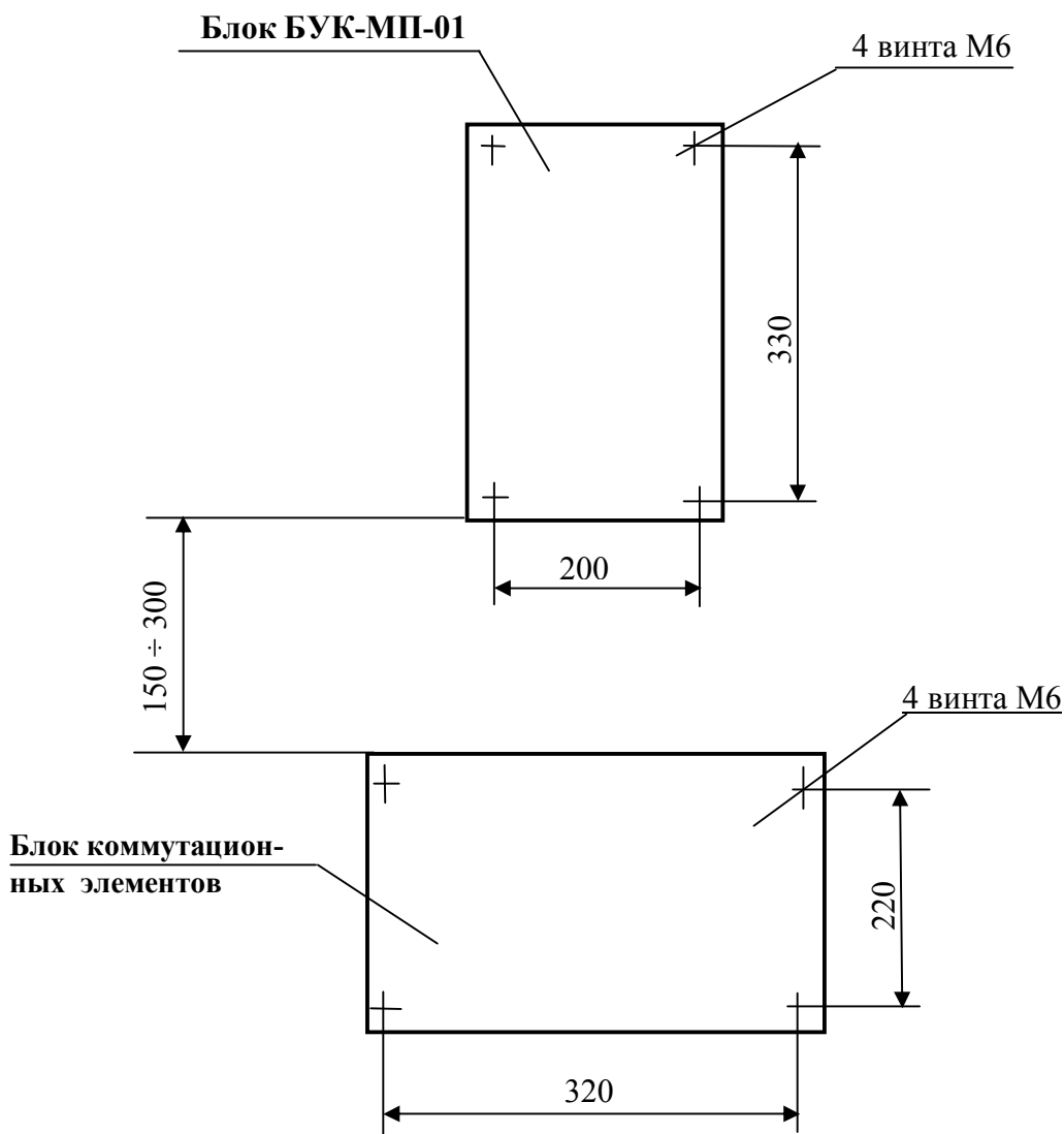
Рис. 1. Разметка под установку блока БУК-МП-01 и блока коммутационных элементов.
